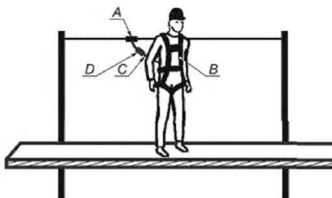
Рисунок 5 — Пример страховочной системы со стропом и амортизатором
