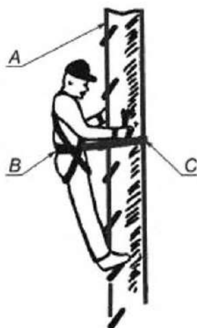
А — крепление; В — привязь; С — стrop для системы позиционирования (применяется для работ на столбах)
