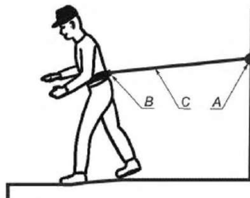
А — анкерная точка, В — привязь; С — строп
