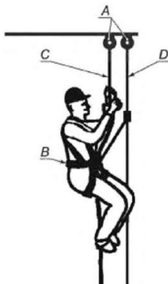
A — анкерная точка; B — привязь; C — рабочий канат; D — страховочный канат
