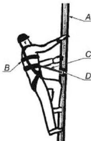
Рисунок 7 — Пример страховочной системы со средством защиты втягивающего типа
