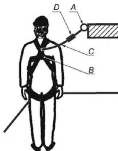
Рисунок 5 — Пример страховочной системы со стропом и амортизатором
